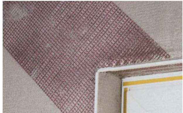
Bild 7: Armierungspfeil an Öffnungsecken
