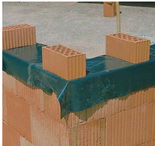
Bild 11: Abdeckung von Mauerkronen
