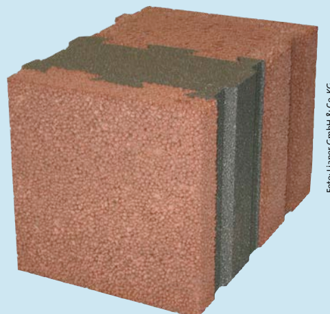
Kombistein mit durchgehender Dämmschicht (Leichtbetonstein)
