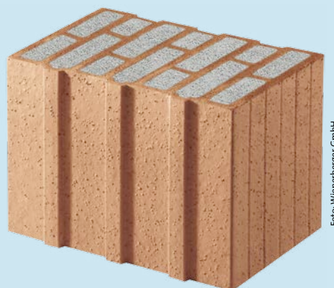
Mit mineralischem Dämmstoff gefüllter hochwärmedämmender Ziegel
