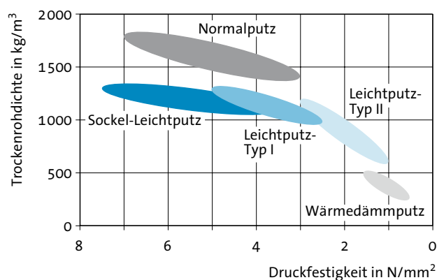
Bereiche für die Trockenrohdichte und Druckfestigkeit üblicher Außenputze (Unterputze)
