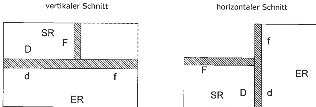
Bild A1: Bezeichnung der Übertragungswege bei versetzten Räumen
