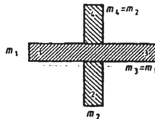
Bild 2: Kreuzstoß mit den in Frage kommenden Übertragungswegen
